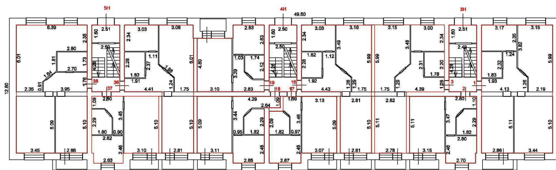
План этажа 1 этаж
