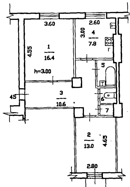
План 4 этажа
